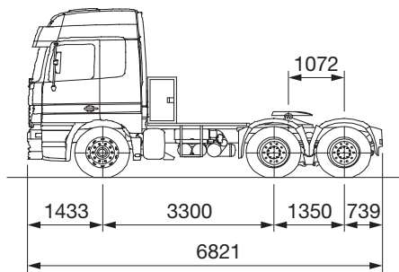
Mercedes-Benz Actros 3353
